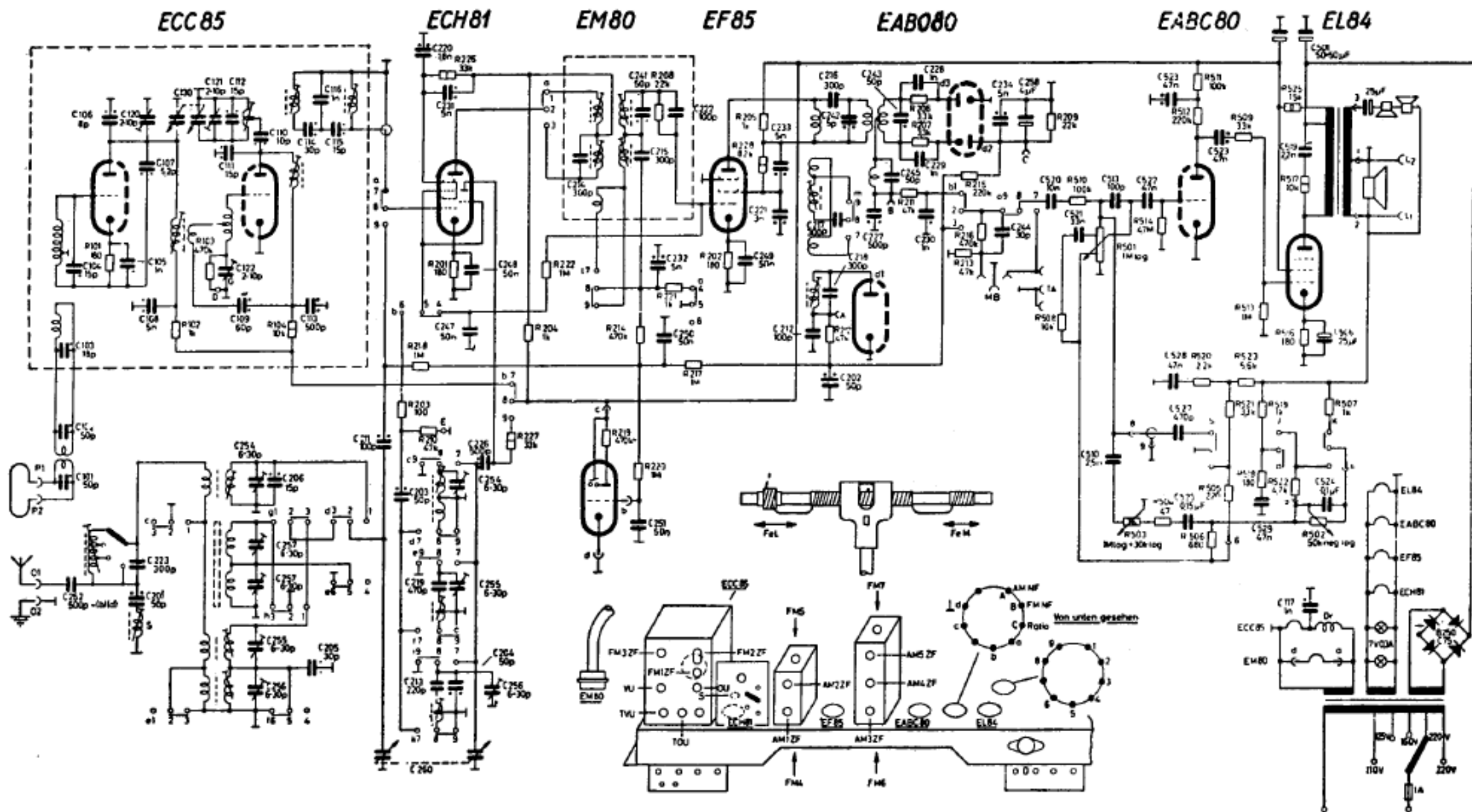
METZ RADIO APPARATEFABRIK (Capriotti) - Mod. AM/FM 212. Onde medie con antenna in ferrite, onde corte e, a modulazione di frequenza, onde ultracorte. Media frequenza AM a 460 kc/s, FM a 10,7 Mc/s. Potenza d'uscita 4 watt indistorti. Consumo 48 watt.
